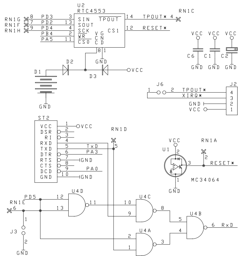
J3 gesteckt schaltet RxD zur CPU durch
